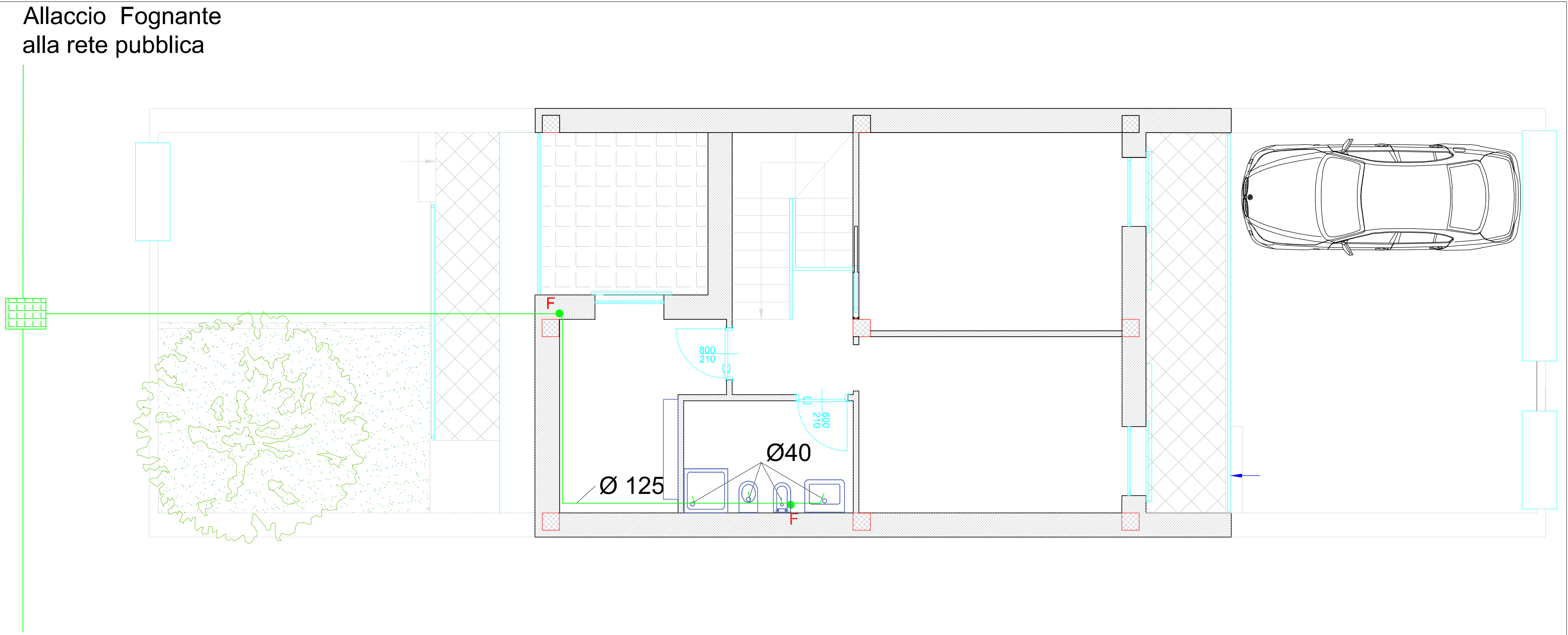
Layout rete di fognatura nera primo piano, scala 1:50
