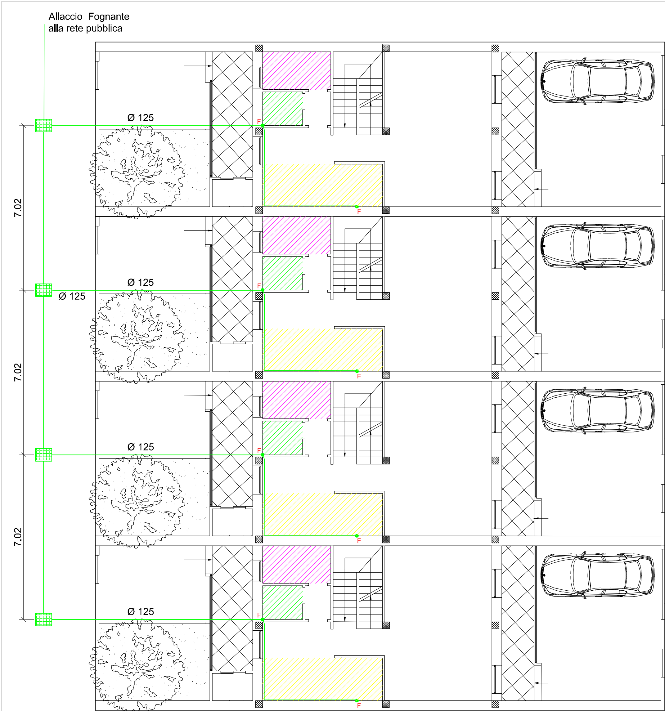
Schema planimetrico della rete di fognatura nera e indicazione dei vani serviti, scala 1:100
