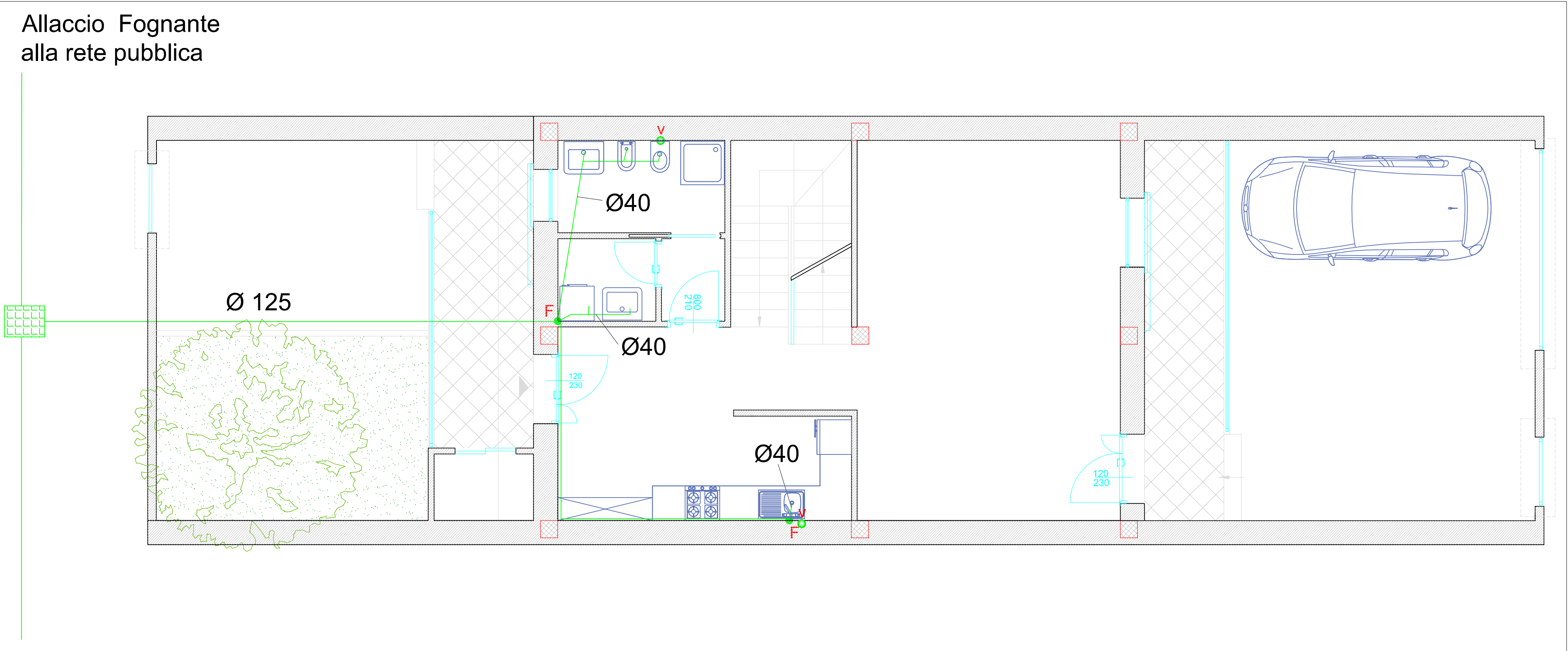
Layout rete di fognatura nera piano terra, scala 1:50
